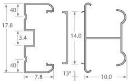
Perfil de Consola Clásica de aluminio extruido (2mm) y acabado con resina epóxica
