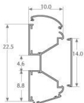
Perfil de Consola 3V Delta de aluminio extruido (2mm) y acabado con resina epóxica
